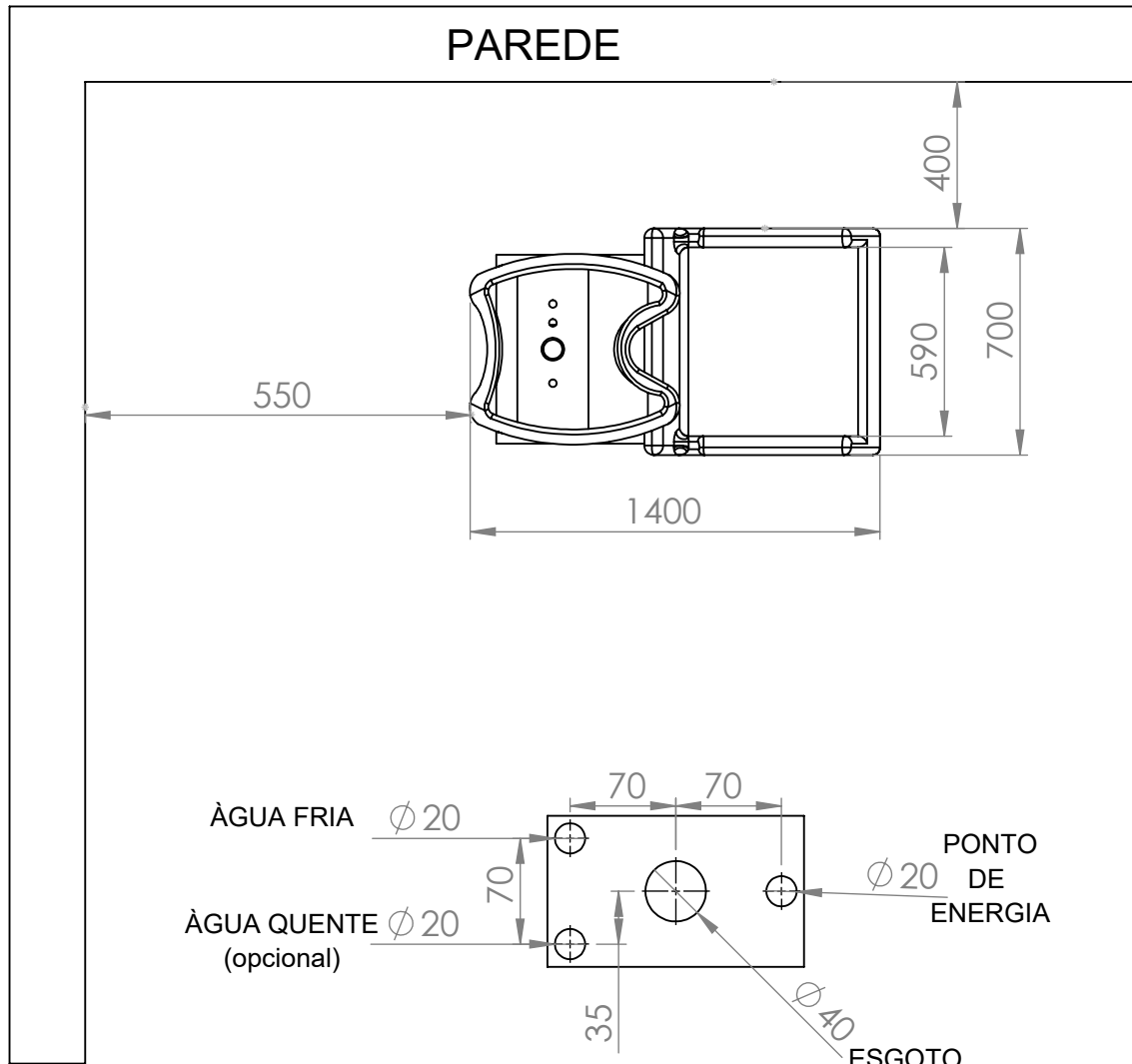
Esquema de instalação (Sob acento)
